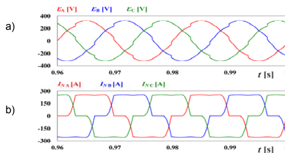
Rys. 6. Przebiegi czasowe prądów i napięć w sieci z dodatkowym obciążeniem w odgałęzieniu i przy rozwartych zaciskach w PCC: a) napięcie sieci; b) prąd sieci
