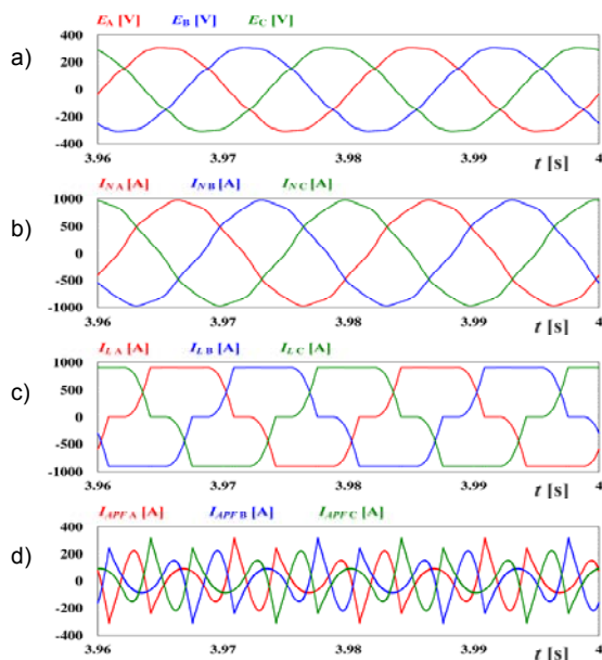
Rys. 4. Przebiegi czasowe prądów i napięć w sieci nierozgałęzionej, przy zastosowaniu klasycznego, równoległego filtra aktywnego: a) napięcie sieci; b) prąd sieci; c) prąd obciążenia; d) prąd kompensatora
