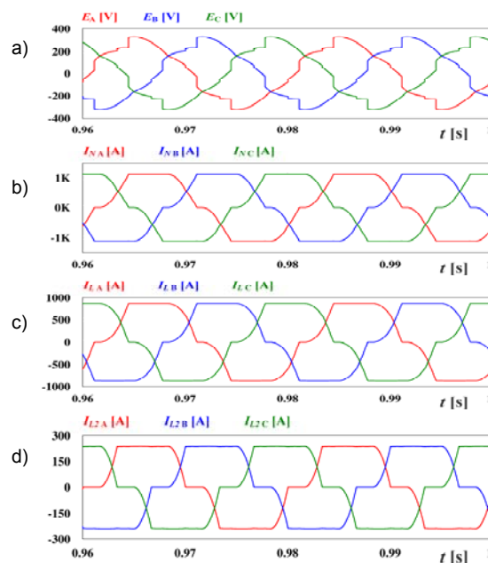
Rys. 7. Przebiegi czasowe prądów i napięć w sieci rozgałęzionej, bez filtra aktywnego: a) napięcie sieci; b) prąd sieci; c) prąd obciążenia NL2 włączonego w PCC; d) prąd obciążenia NL1 włączonego przed PCC
