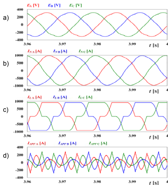
Rys. 5. Przebiegi czasowe prądów i napięć w sieci nierozgałęzionej, przy zastosowaniu napięciowego, równoległego filtra aktywnego: a) napięcie sieci; b) prąd sieci; c) prąd obciążenia; d) prąd kompensatora
