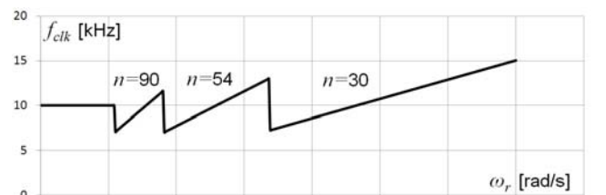
Rys.7. Wykres częstotliwości sterowania f_{clk} w funkcji prędkości obrotowej mechanicznej wirnika \omega_r
